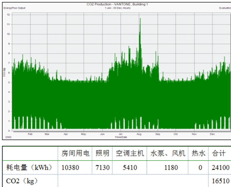
图表 3 DB 模拟结果——CO 2 产生量
